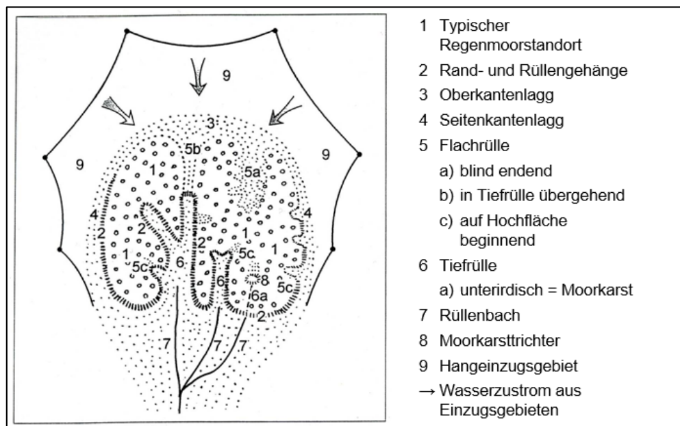
Abbildung KBS 5 Hydromorphologische Strukturelemente eines idealisierten erzgebirgischen Hang-Regenmoores (KÄSTNER & FLÖßNER 1933, verändert EDOM 2001)
