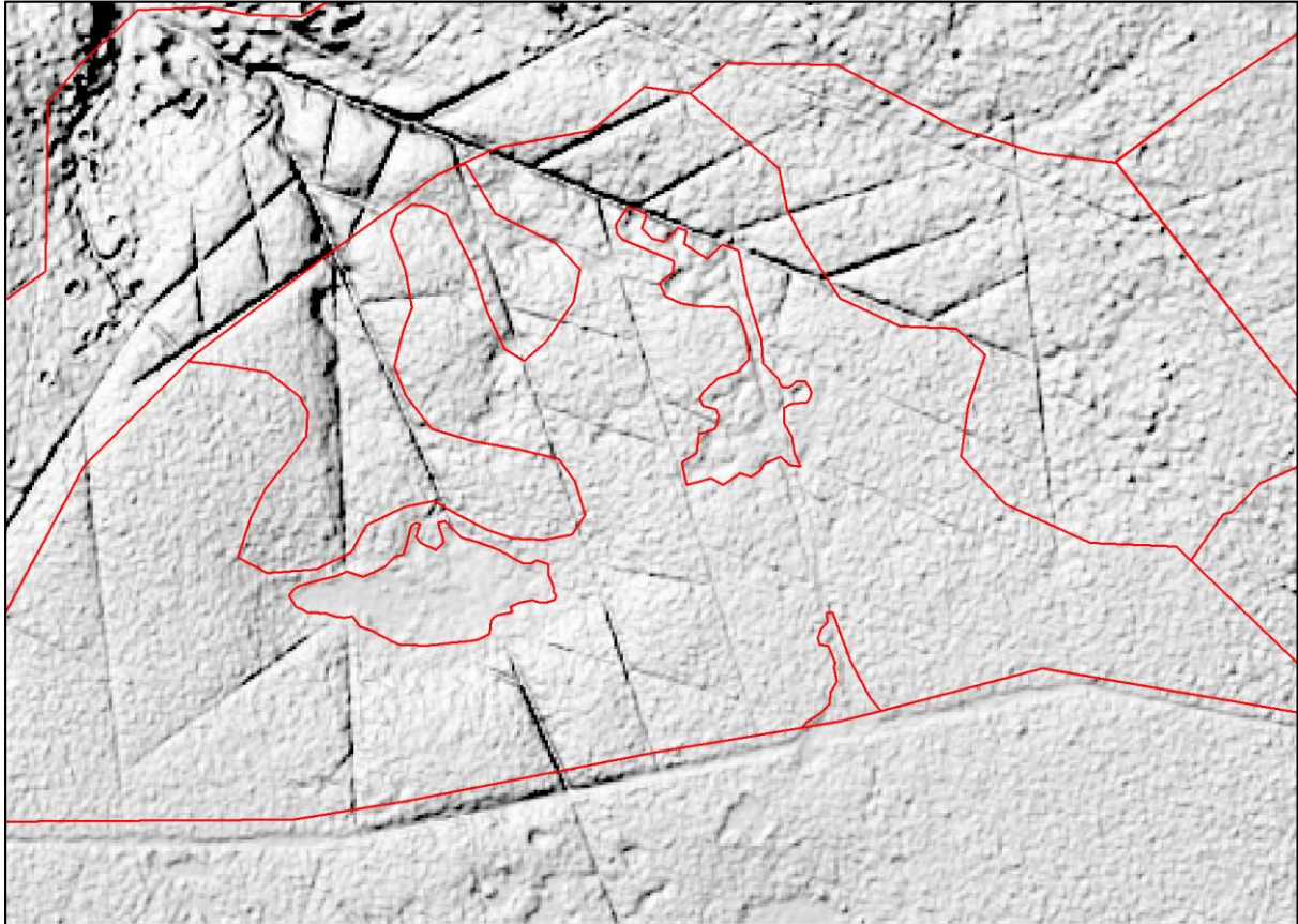
Abbildung 3 Beispiel eines digitalen Geländehöhenmodells. Zu erkennen sind Entwässerungsgräben, die zur Orientierung und LRT-Abgrenzung dienen können (Großer Kranichsee).
